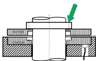
スクリューマウントロータ
