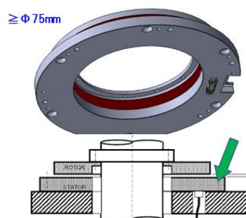
外周マウントステータ
